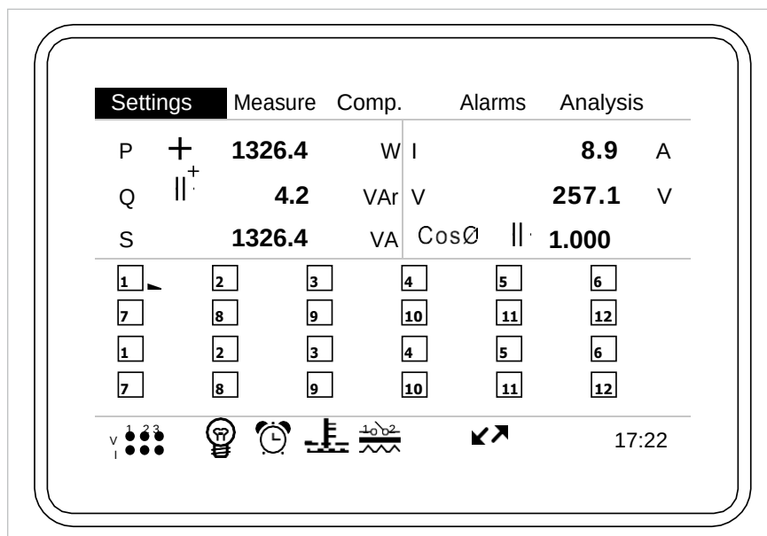
Fig. 1-3 Powersave Pro con 24 RELÉS
