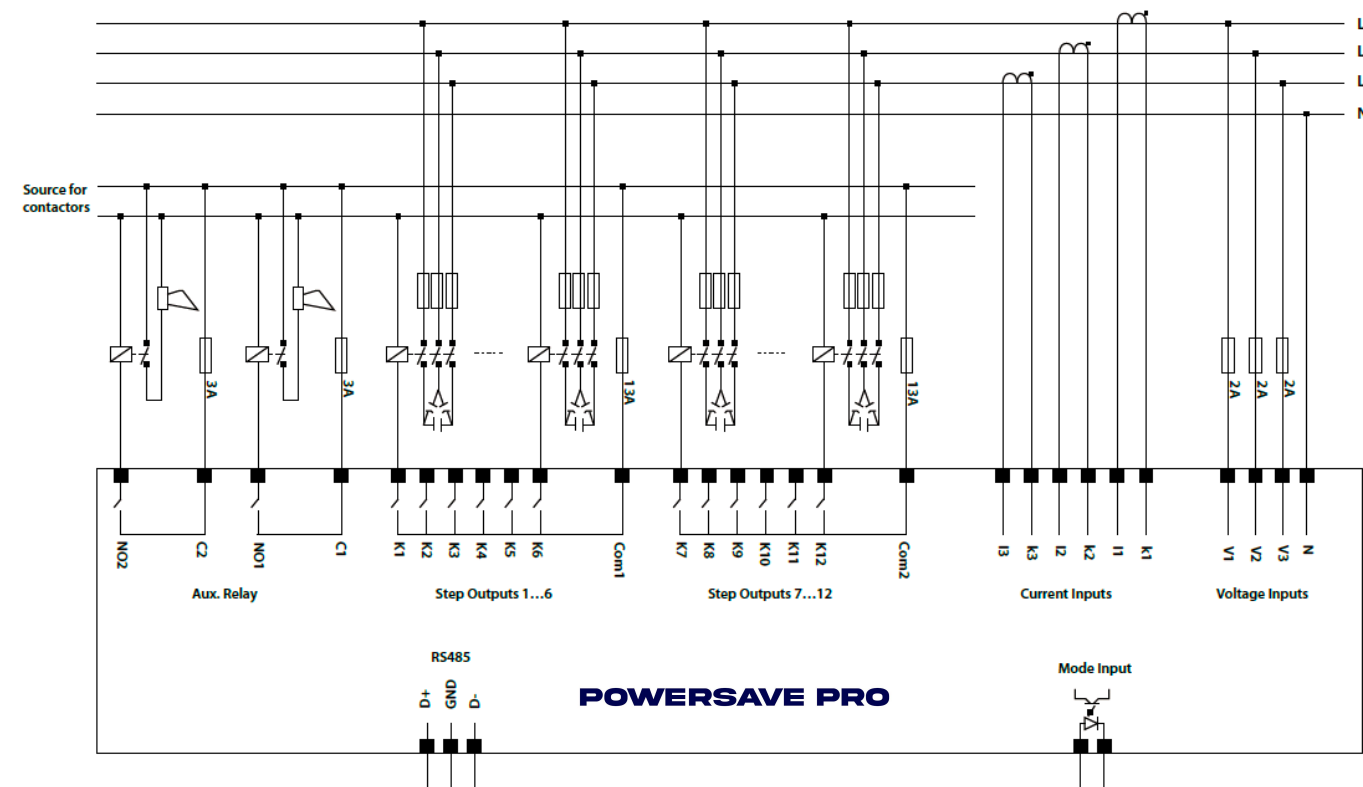
Fig. 2-6 Diagrama de conexión Powersave Pro (12 Steps)
