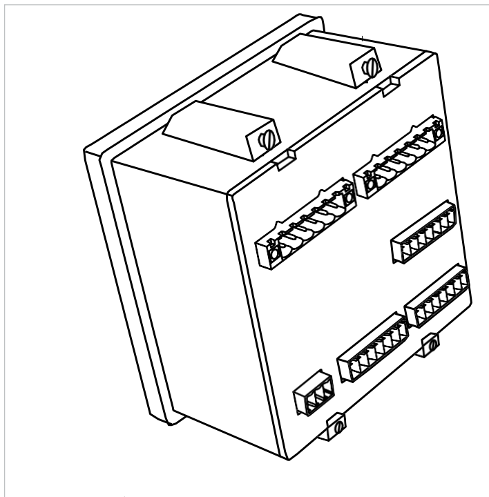
Fig. 2-2 Asegurando Powersave Pro
