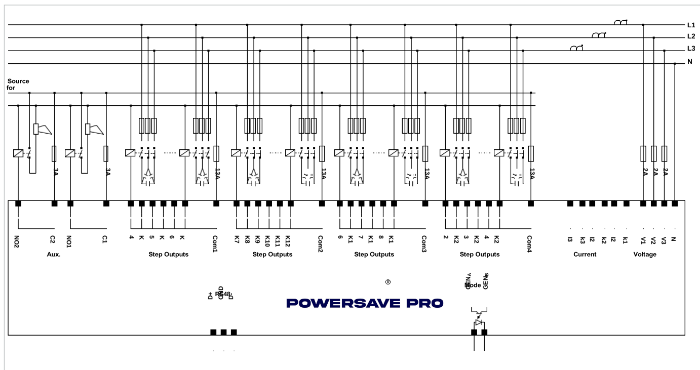
Fig. 2-7 Diagrama de conexión Powersave pro (24 Steps)
