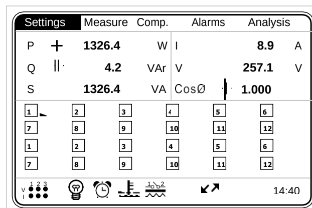
Fig. 3-32 Powersave Pro con 24 Relés
