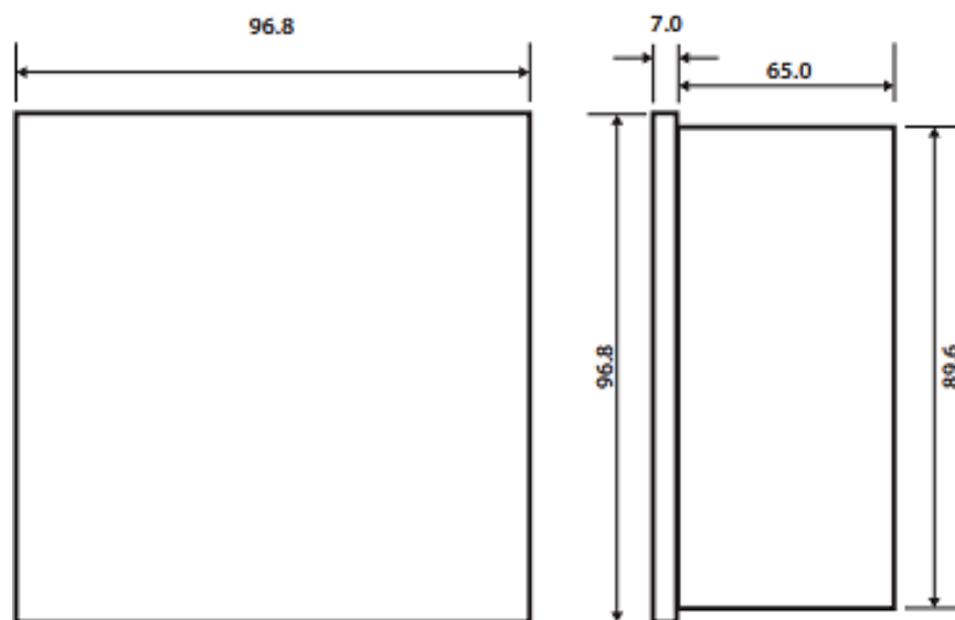
Figura 2. Dimensiones
